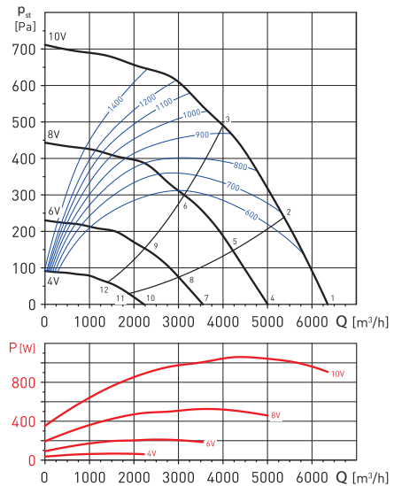
KABB-6000/450 Ecowatt
