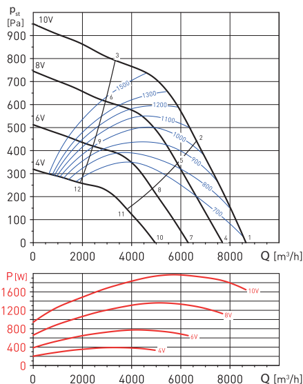
KABT-9000/500 Ecowatt
