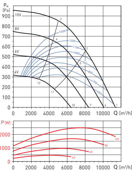
KABT-12000/560 Ecowatt
