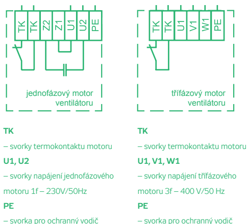
OBRÁZEK 5 – SCHÉMATA ZAPOJENÍ
