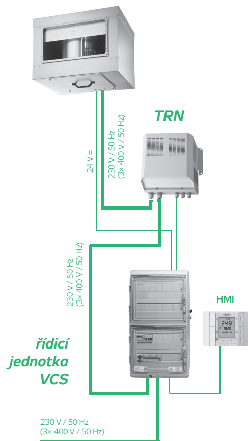
OBRÁZEK 8 – ZAPOJENÍ VENTILÁTORŮ
