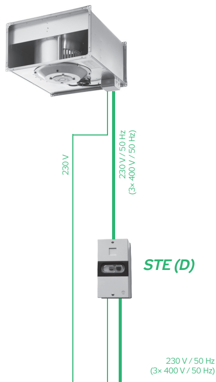
OBRÁZEK 7 – ZAPOJENÍ VENTILÁTORU
