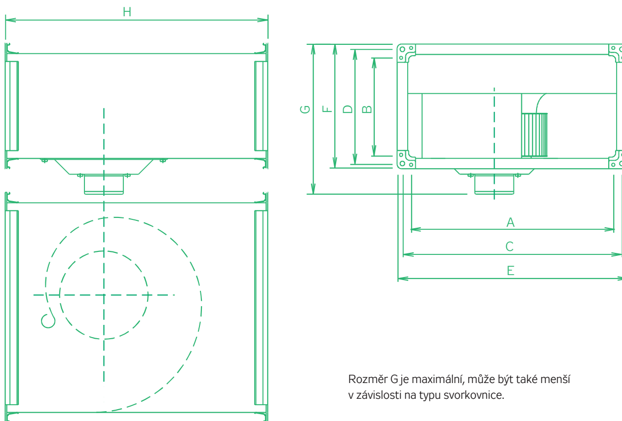
OBRÁZEK 5 – ROZMĚRY VENTILÁTORŮ
