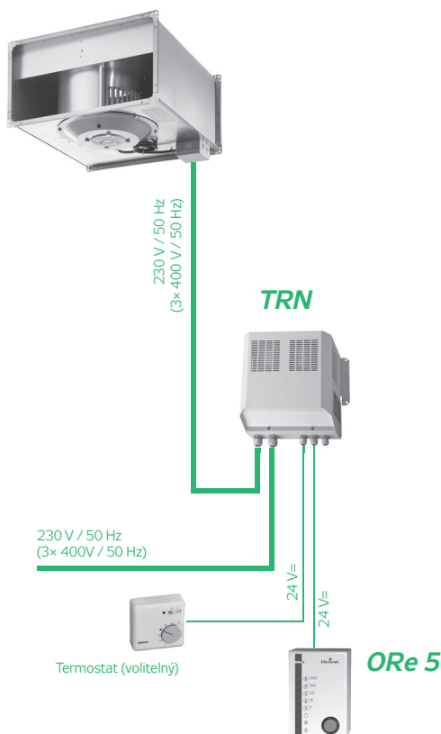
OBRÁZEK 8 – ZAPOJENÍ VENTILÁTORU
