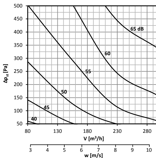
Graf č. 4 Hladina akustického výkonu L_{WA} [dB(A)] vyzářeného do potrubí DN160
