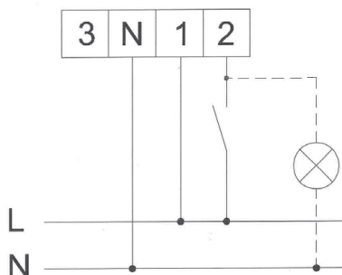
obr. 7 - schéma zapojení
