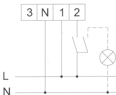
schéma zapojení - je nutné použít dvoupólový vypínač
